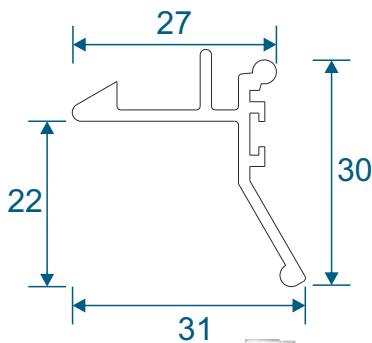
SG57- Sprung Handle
